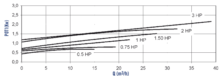
Courbes de puissance-débit Power-Flow Curves
